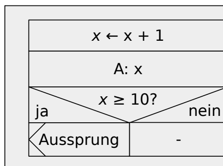
Abb. 53: Struktogramm: Endlosschleife mit Aussprung
