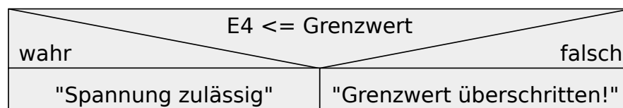
Abb. 30: Fallunterscheidung
