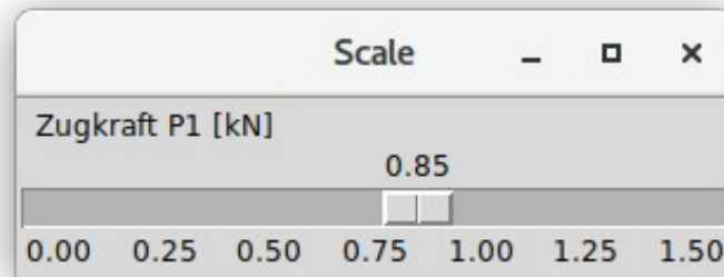
Abb. 119: Horizontales Scale-Widget
