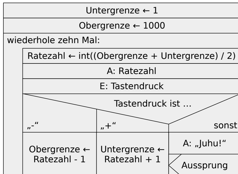
Abb. 54: Struktogrammbeispiel „Zahlenraten“
