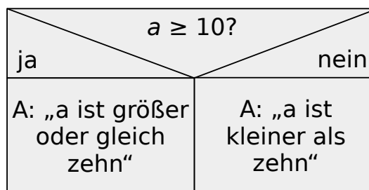
Abb. 48: Struktogramm: Fallunterscheidung
