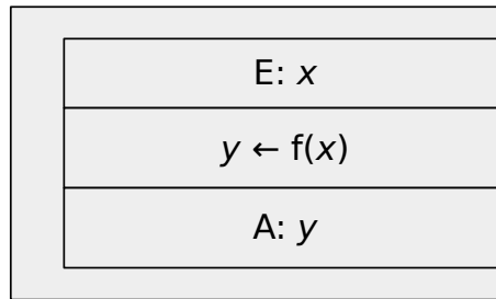
Abb. 52: Struktogramm: Endlosschleife
