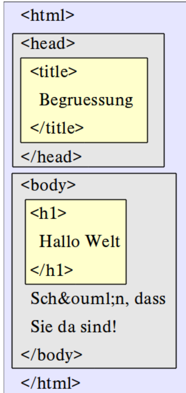
Abb. 43: HTML-Struktur
